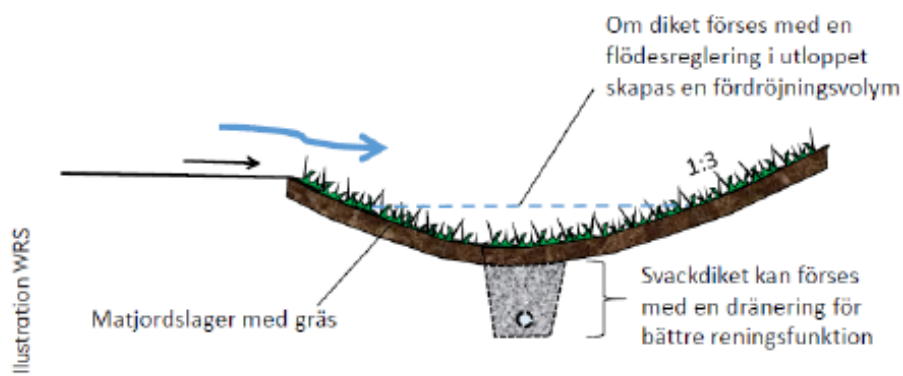
Figur 20 Principskiss för ett svackdike. Svackdiken etableras på naturmark i nivå under ytan som ska avvattnas. Reningsfunktionen kan förstärkas genom att anlägga ett dräneringslager med dräneringsledning i botten
